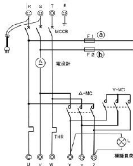
<電動機起動盤主回路図>
