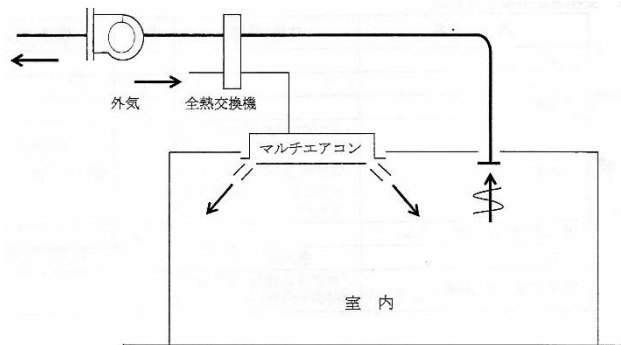
＜空気調和概念図＞
